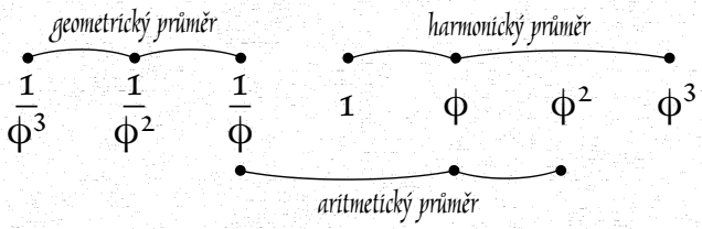
ZLATÁ POSLOUPNOST zahrnuje všechny tři průměry čtyř členů
