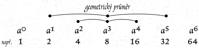
GEOMETRICKÁ POSLOUPNOST obrázek ukazuje, jak se určuje geometrický průměr členů geometrické posloupnosti
