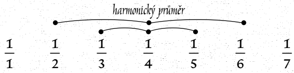
HARMONICKÁ POSLOUPNOST obrázek ukazuje, jak se určuje harmonický průměr členů harmonické posloupnosti
